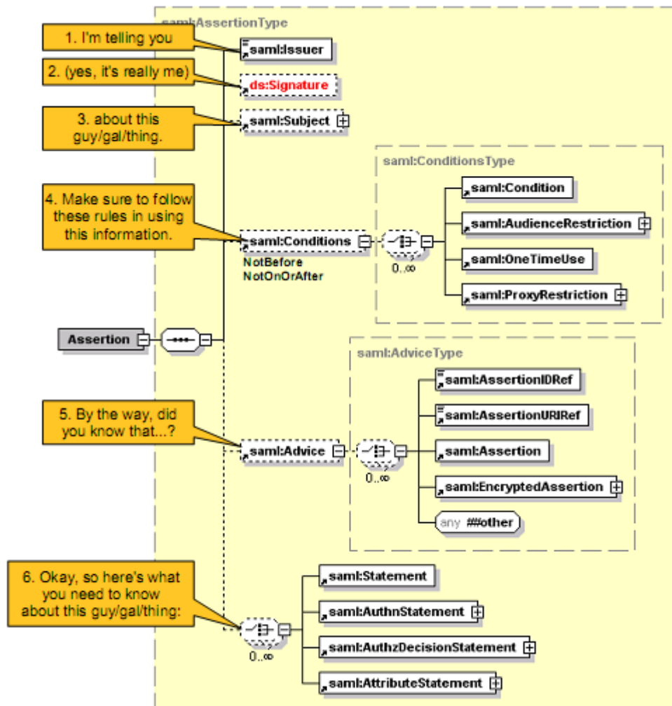
Abbildung 40: Aufbau einer SAML Assertion (aus [Maler06]).
