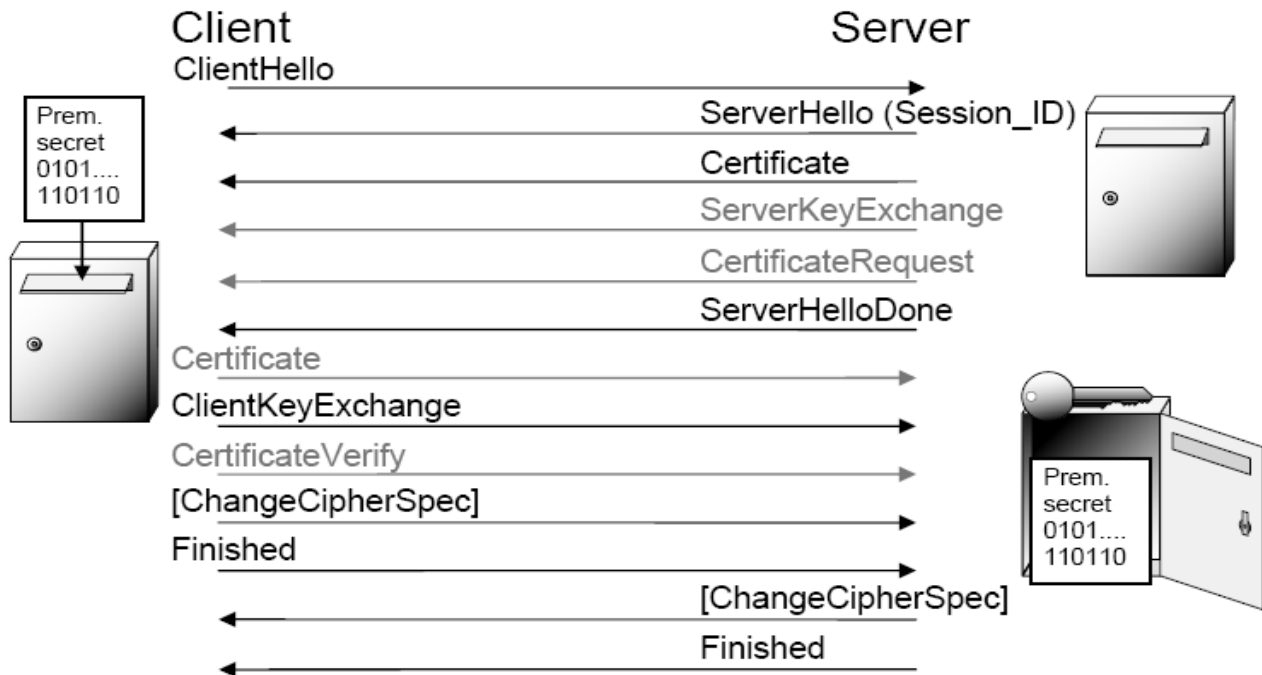
Abbildung 35: Das SSL/TLS Handshake-Protokoll
