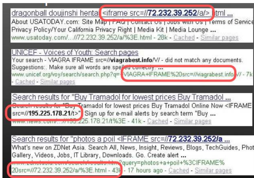
Abbildung 19: Ergebnis spezieller Google-Suchanfragen im Zusammenhang mit der IFrame-Verseuchung diverser Webseiten.
