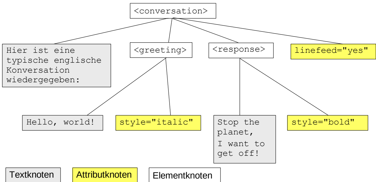
Abbildung 36: Darstellung des XML-Dokuments aus Tabelle 1 als DOM-Baum
