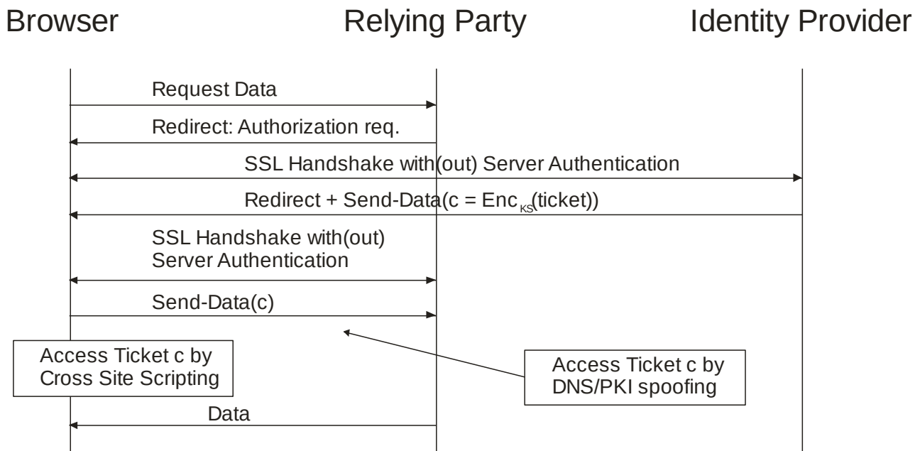
Abbildung 42: Sicherheitsprobleme eines generischen Single-Sign-On-Protokolls
