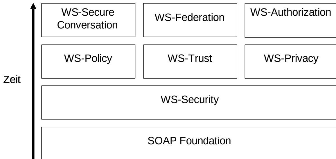
Abbildung 39: Die IBM/Microsoft-Roadmap zur Absicherung von Webservices.
