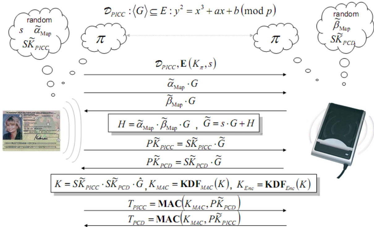
Abbildung 45: Ablauf des PACE-Protokolls [BSI-TR-03112-7]
