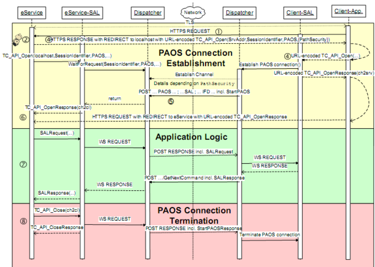
Abbildung 44: Gesamtüberblick Verbindungsaufbau (aus [BSI-TR-03112-7]).
