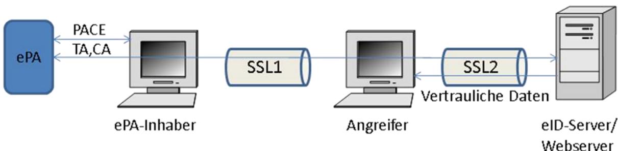
Abbildung 50: Man-in-the-Middle-Angriff auf die SSL-Verbindung
