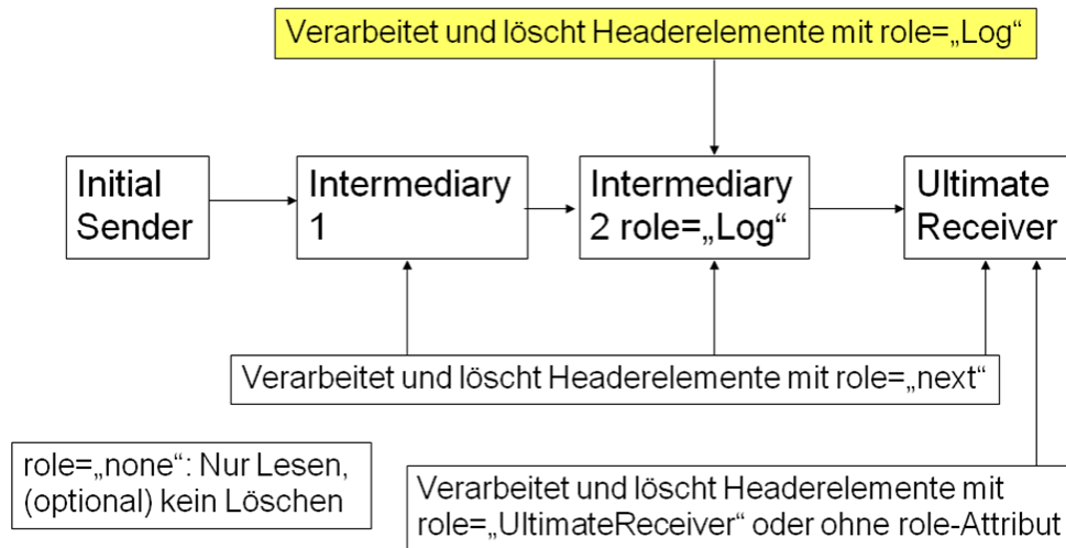
Abbildung 38: Das "role"-Attribut zur Steuerung der SOAP-Kommunikation über mehrere beteiligte Instanzen.
