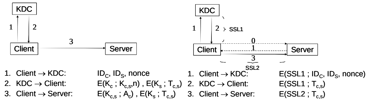
Abbildung 41: Gegenüberstellung von Kerberos und einem Web-basierten Single-Sign-On-Protokoll.
