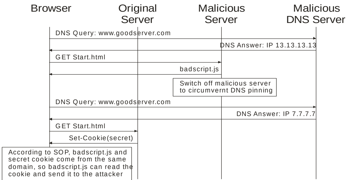
Abbildung 23: Dynamic Pharming-Angriff zum Diebstahl von Identitätsdaten
