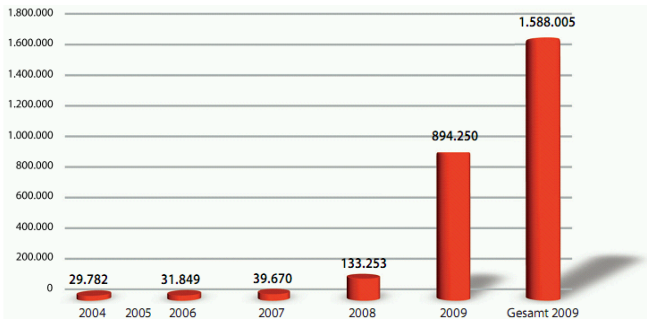
Abbildung 24: Anzahl neuer Malware-Samples pro Jahr. (Quelle: GData)
