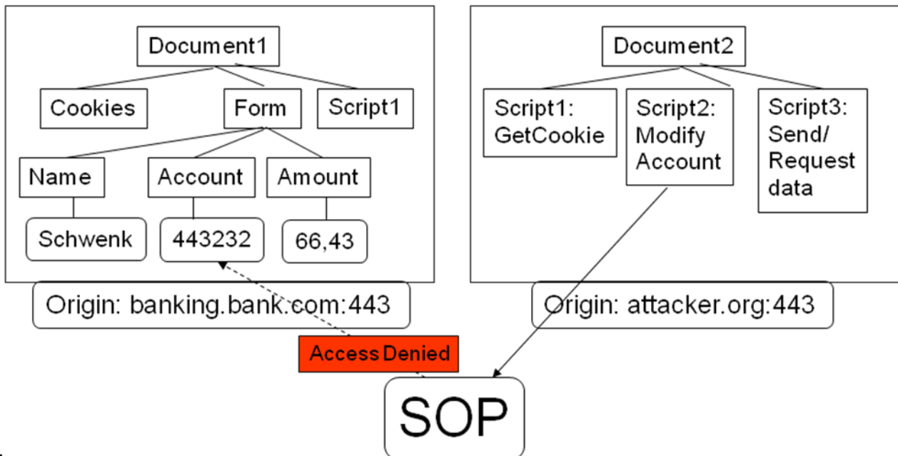
Abbildung 34: Funktionsweise der Same Origin Policy.
