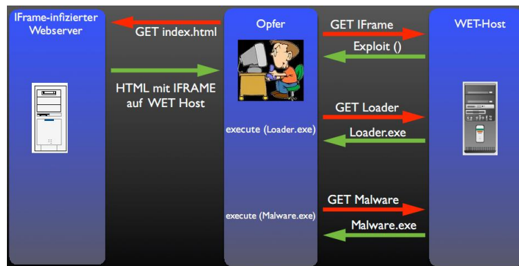
Abbildung 20: Schrittfolge eines WET-Angriffs.
