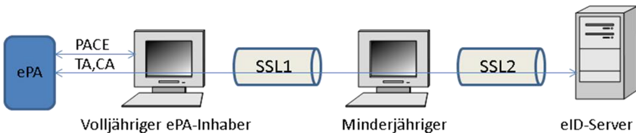
Abbildung 49: Altersverifikationsproxy zur Umgehung der Altersverifikation
