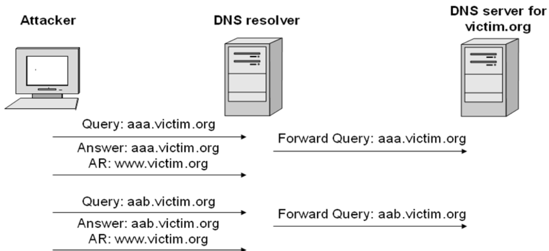
Abbildung 22: Der Kaminski-Angriff auf das Domain Name System
